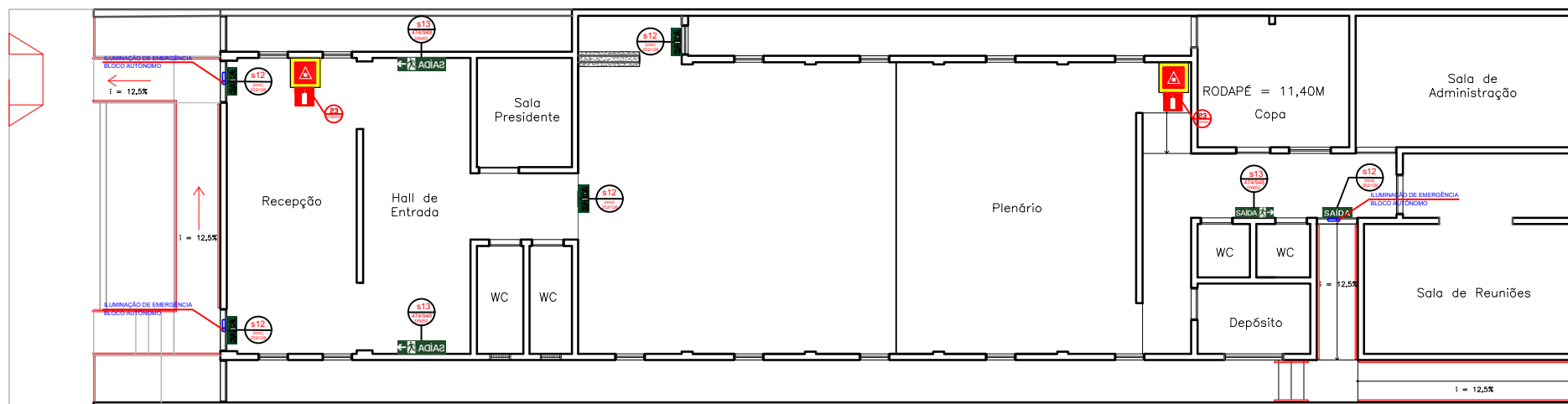
01 Planta Acessibilidade e Combate a incêndio PAV. TÉRREO esc.: 1/75
