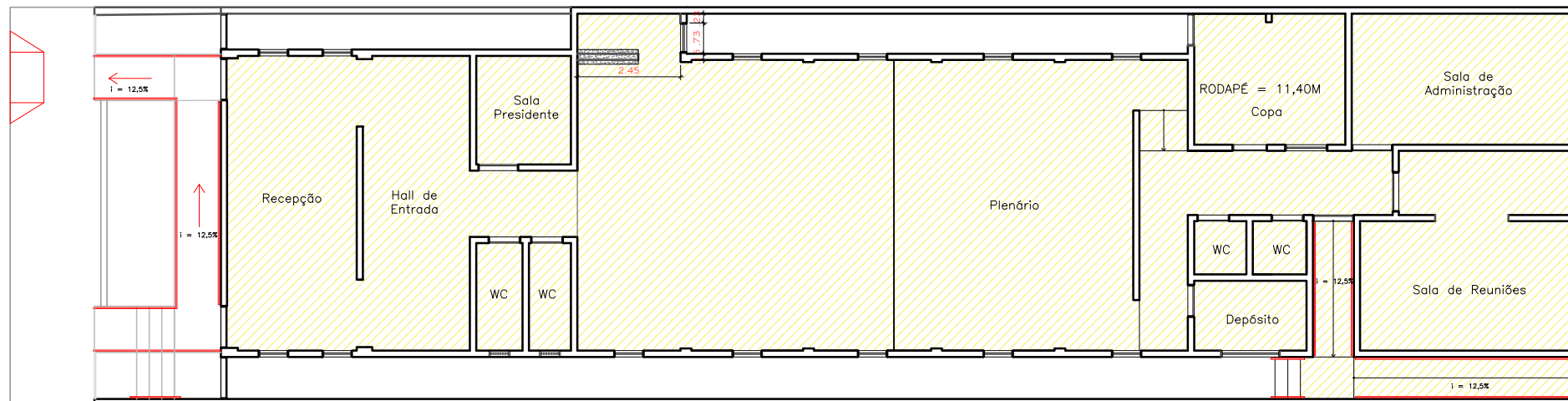
01 Planta de Reforma PAV. TÉRREO esc.: 1/75
